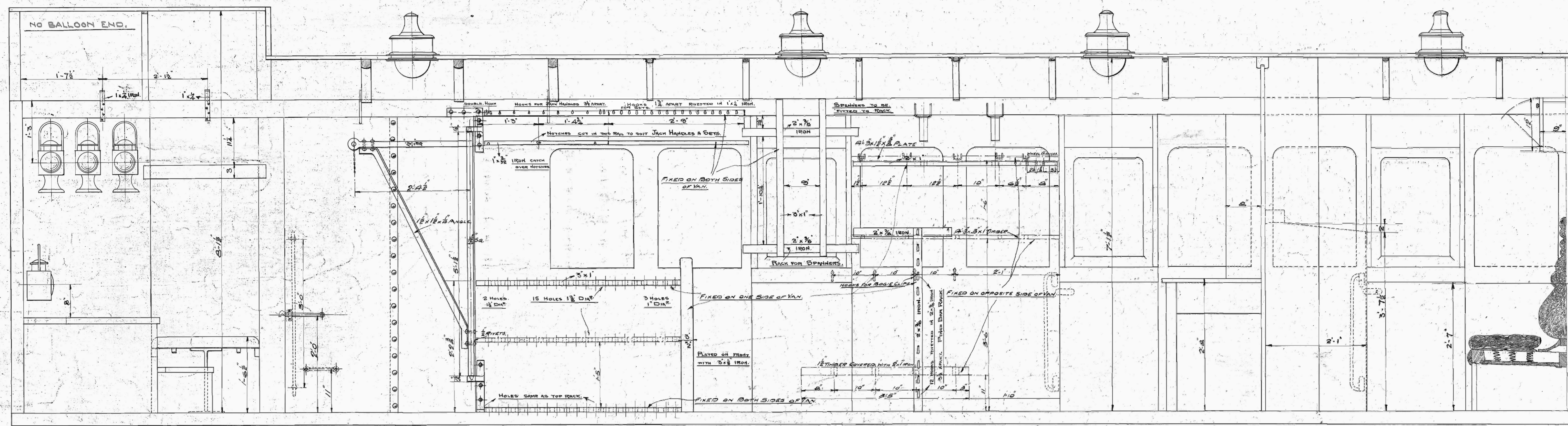
LONGITUDINAL SECTION
