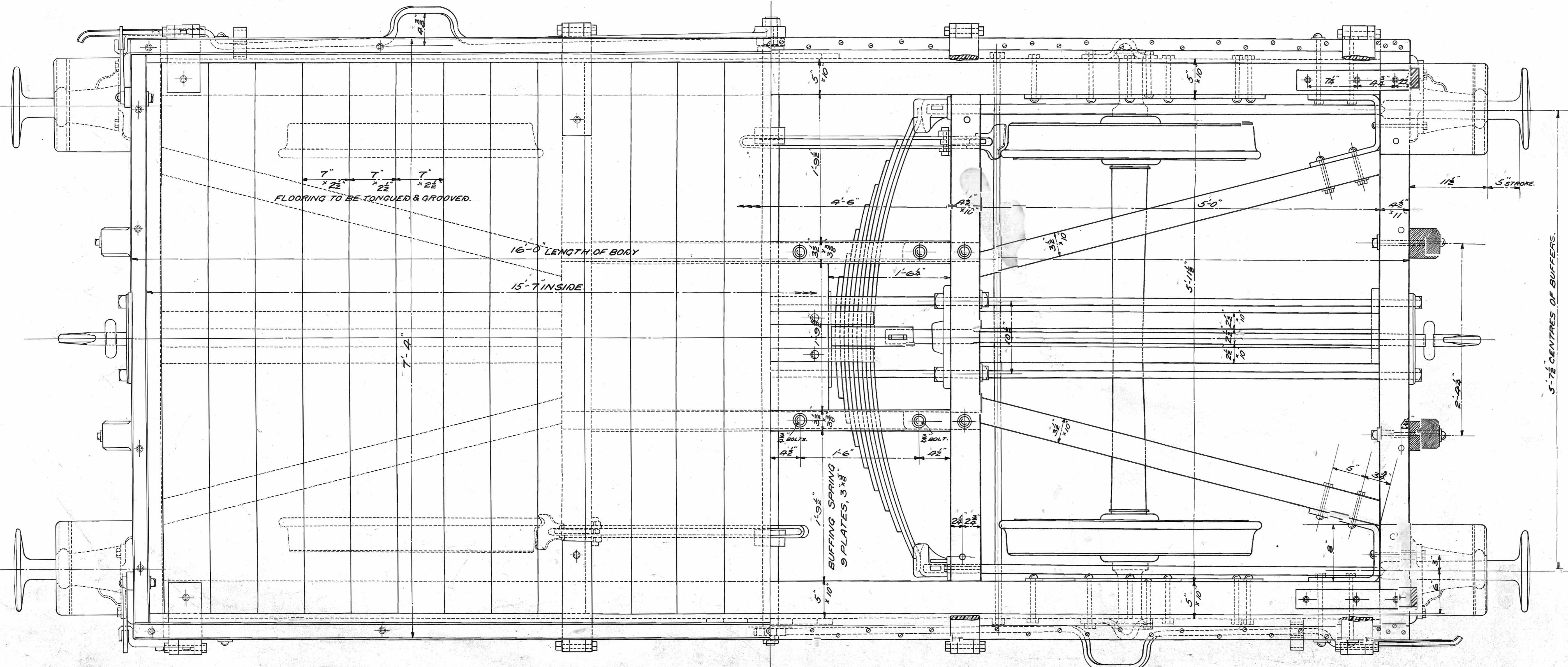
PLAN.
